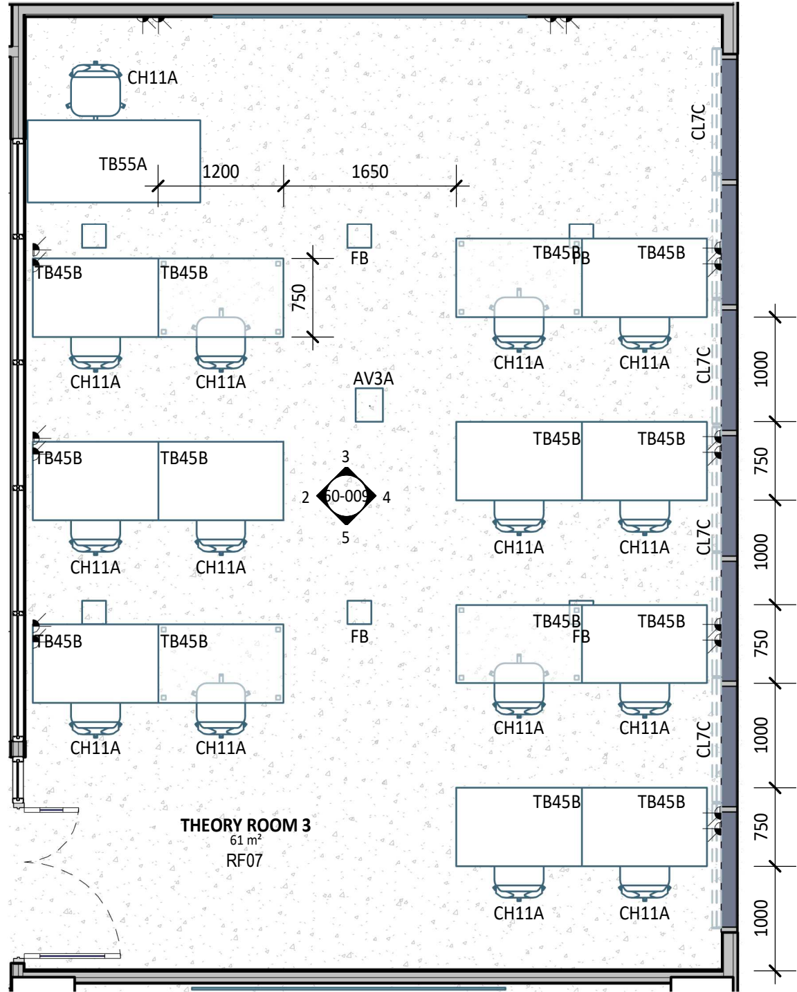
1 PLAN DETAIL 30-01 1 : 50
